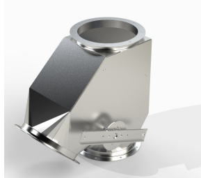
2 Way Y Flipper Valve
